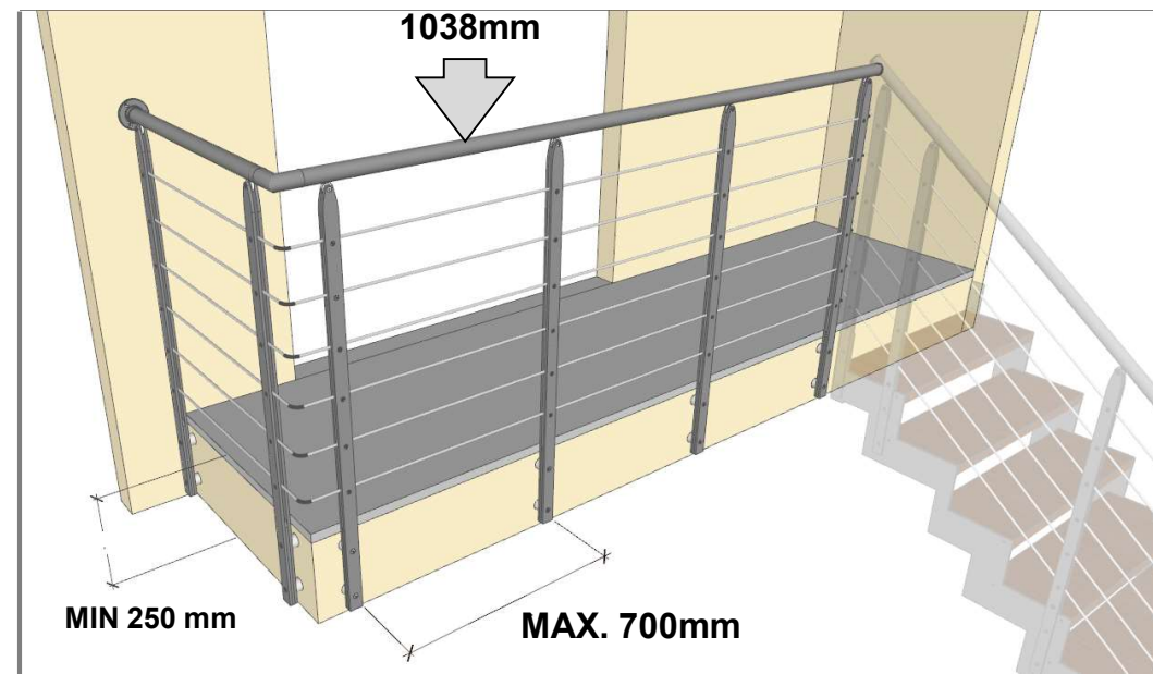
Balaustra con fissaggio a soletta,
