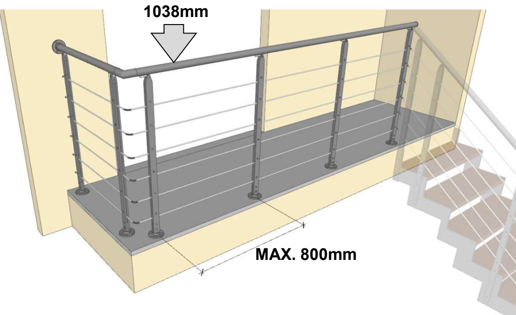
Balaustra con fissaggio a pavimento,
